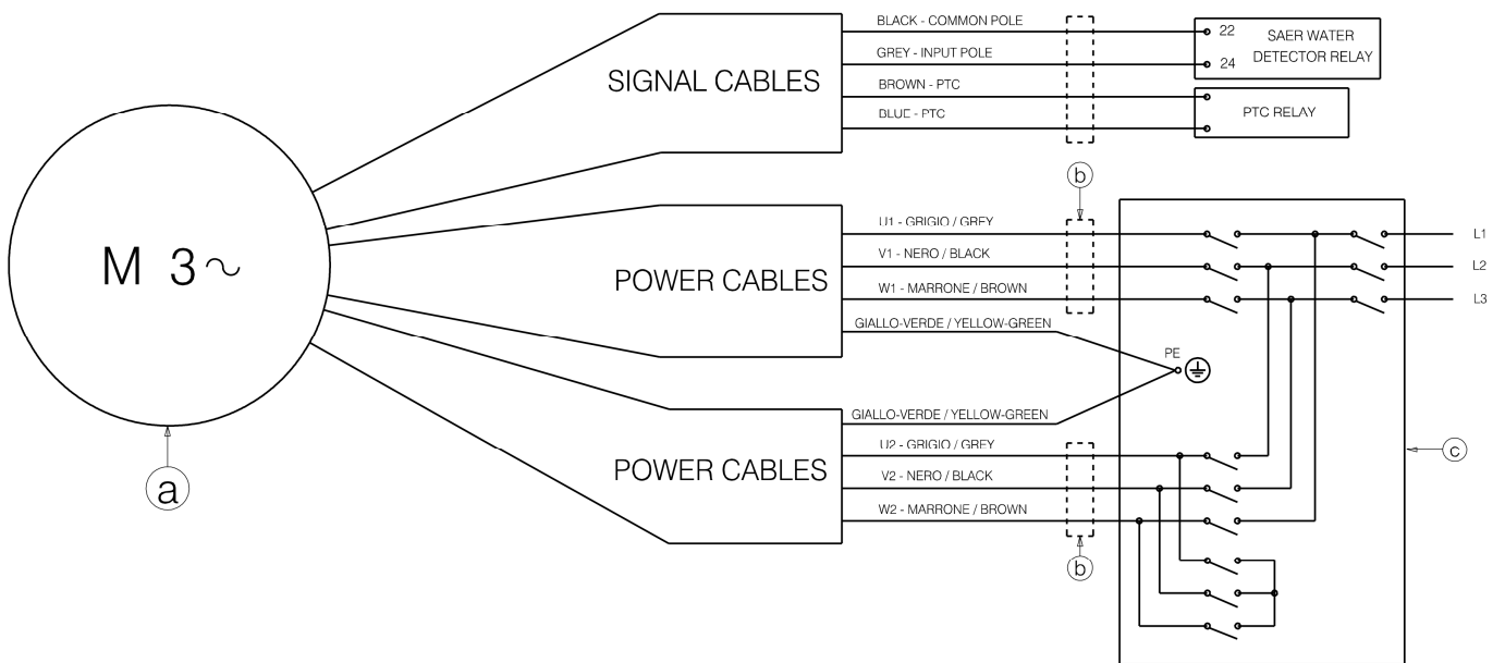
a: Motore / Motor - b: Eventuale giunzione esterna / Possible external junction - c: Quadro di comando / Control panel
