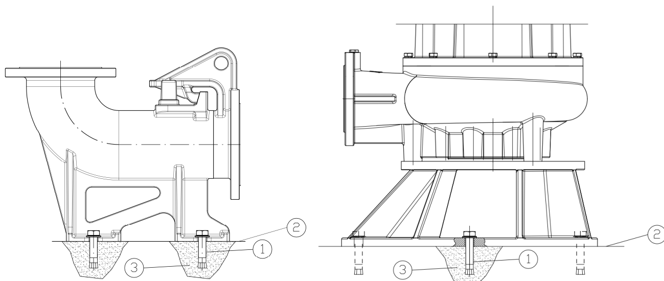
FIG. 5 FISSAGGIO AL SUOLO • GROUND FIXING
