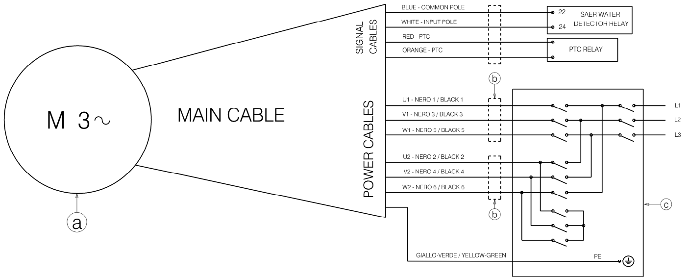
a: Motore / Motor - b: Eventuale giunzione esterna / Possible external junction - c: Quadro di comando / Control panel
