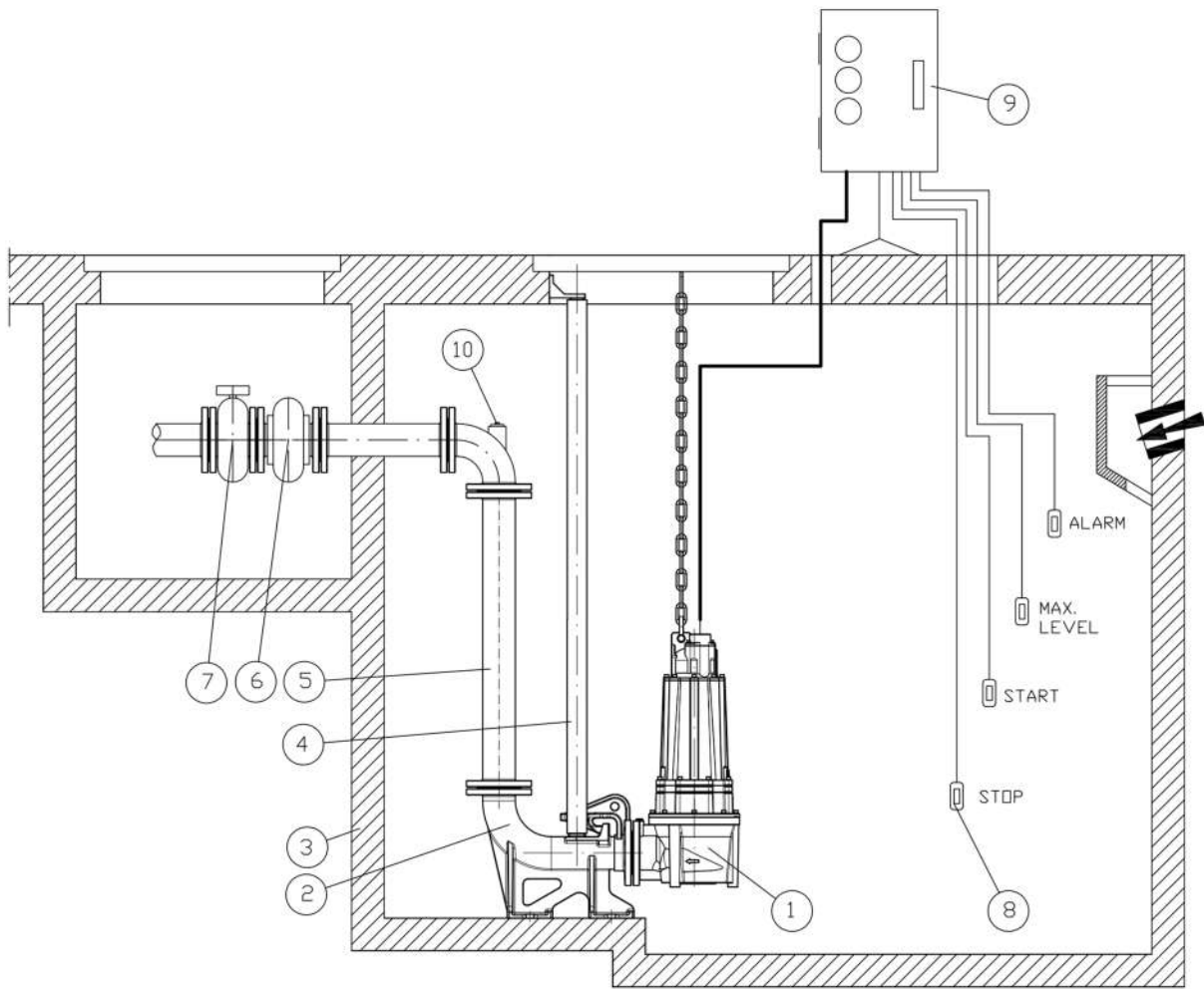
FIG. 4b SCHEMA DI INSTALLAZIONE TIPICO • TYPICAL INSTALLATION DIAGRAM
